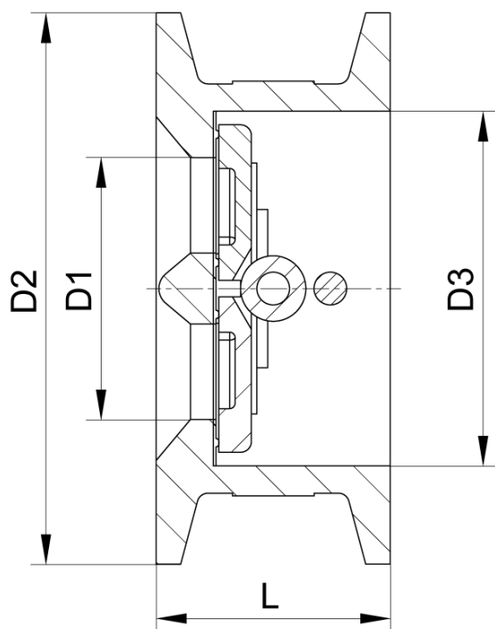
Coupe A-A
