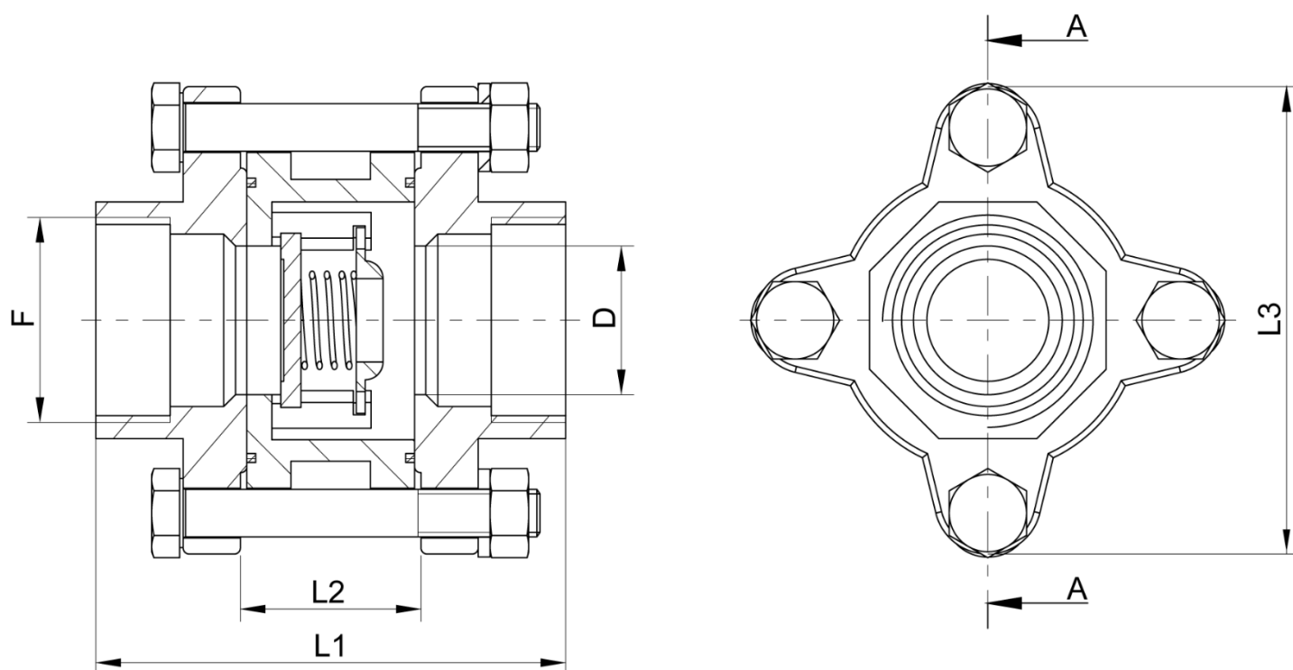
Sección A-A
