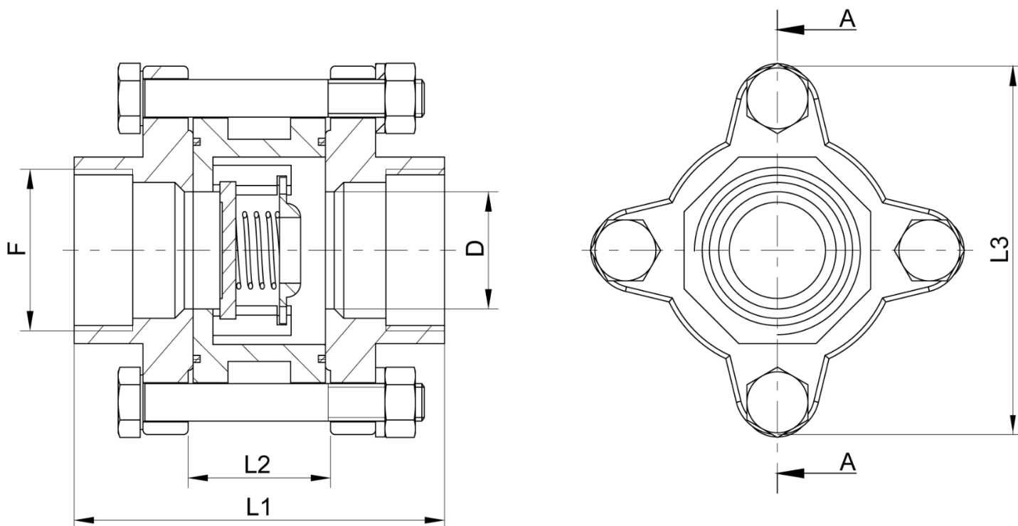
Sección A-A
