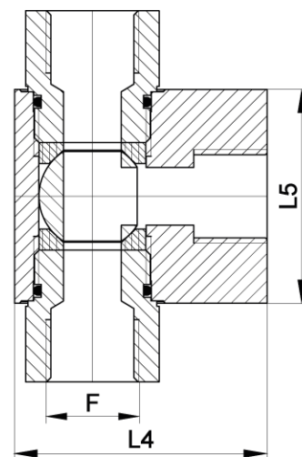
Coupe B-B
