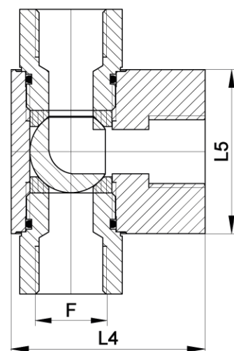
Coupe B-B
