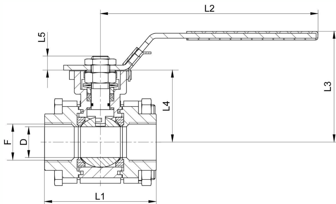
Coupe A-A
