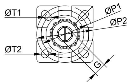
Platine ISO
