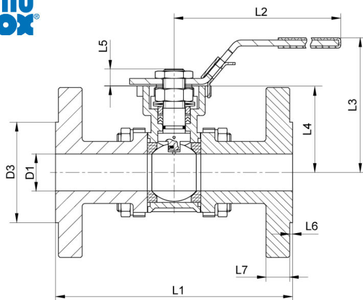
SECCIÓN A-A
