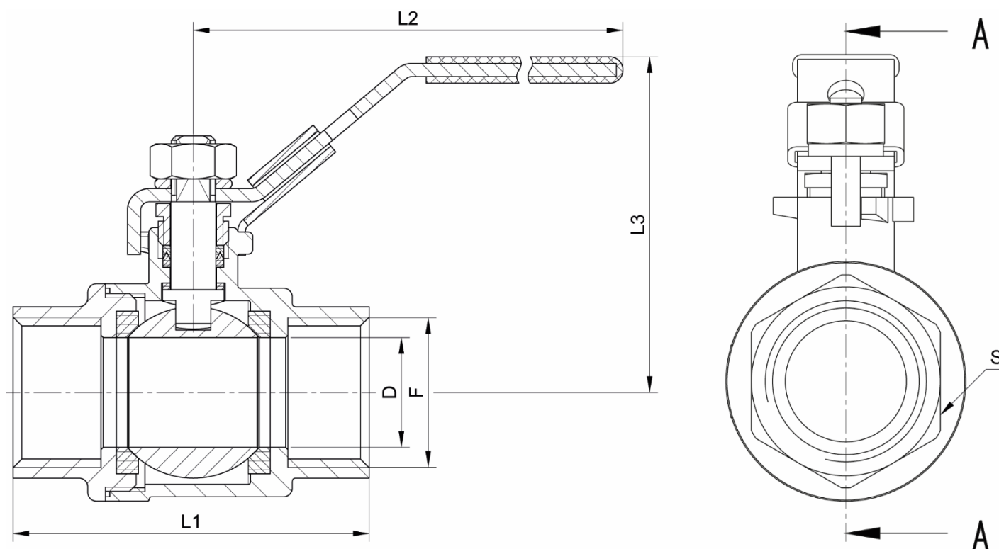
SECCIÓN A-A
