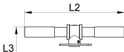
Poignée DN65 - 100 (2"1/2 - 4")
