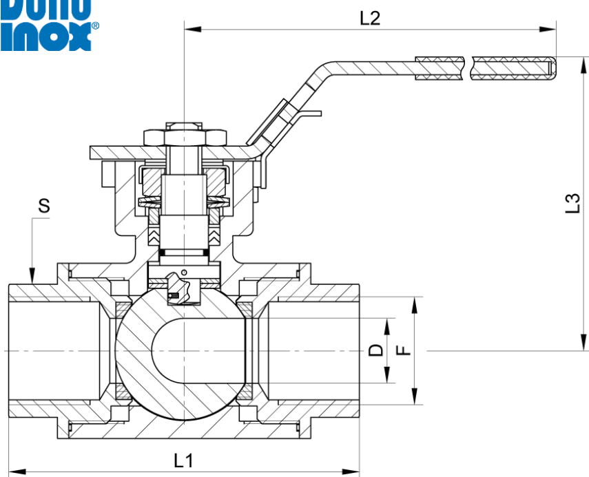
SECCIÓN A-A
