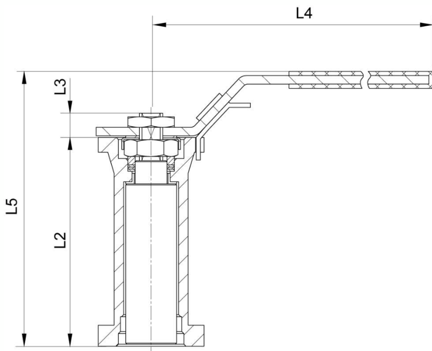
Coupe A-A
