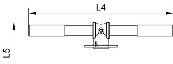
Poignée DN65 à DN150 (2"1/2 à 6")
