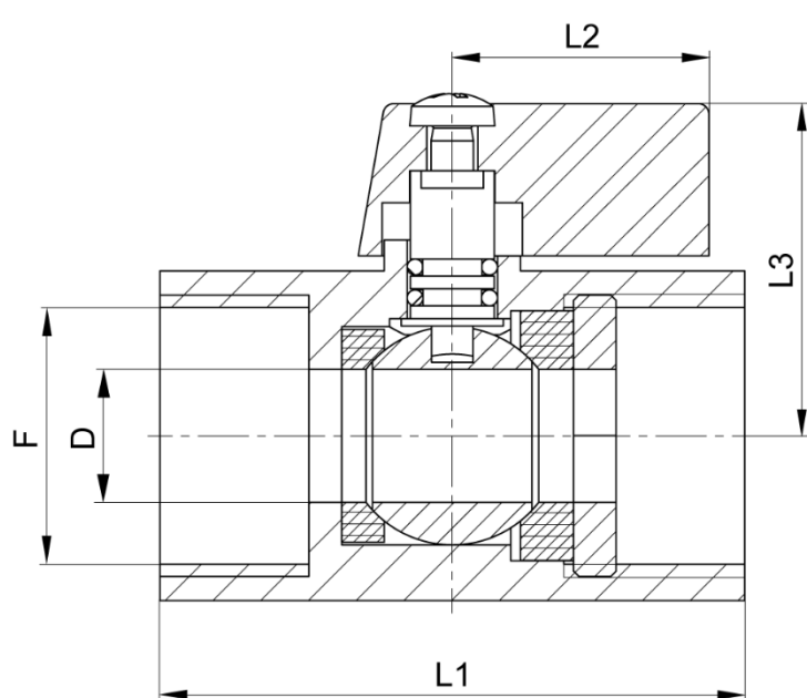
Coupe A-A
