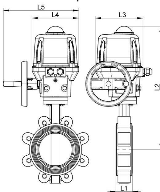
DN125 para DN200
