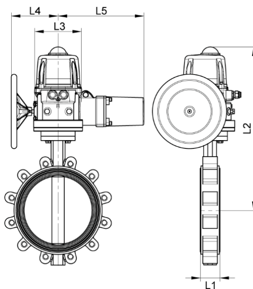
DN250 para DN300
